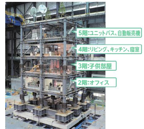
超高層建物の長周期地震動によるオフィス空間などの安全確保を検証する実験 http://www.bosai.go.jp/hyogo/research/movie/movie-detail.html#15 動画:独立行政法人 防災科学技術研究所 E-ディフェンス
