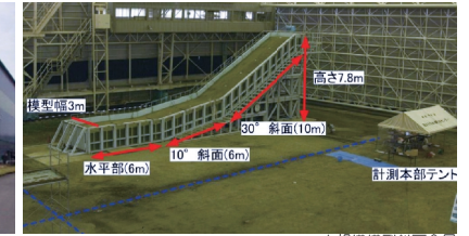
大規模模型斜面全景
